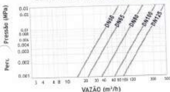
Curva de Perda de Cargas
